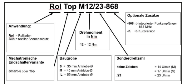
Fig. 13 RevoLine Bezeichnungserklärung
