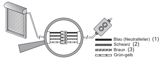
Fig. 6 Anschluss für Montagekabel
